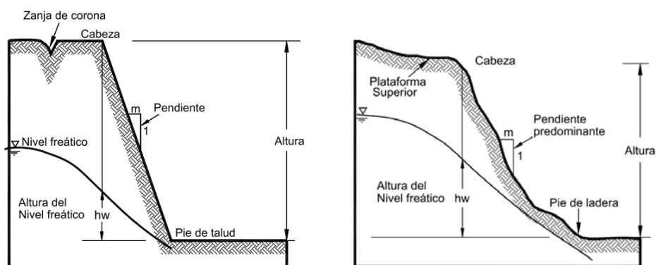
Figura 1. Partes que componen un talud o una ladera: a) Talud (conformado antropicamente), y b) Ladera natural [9]
