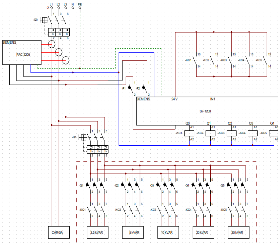
Figura 19. Esquema eléctrico
