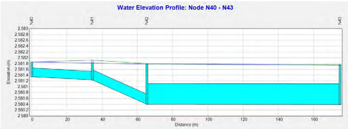
Figura 13. Perfil de los tramos y pozos desde el N40 al N43 del barrio Isla del Sol para el caso 4
