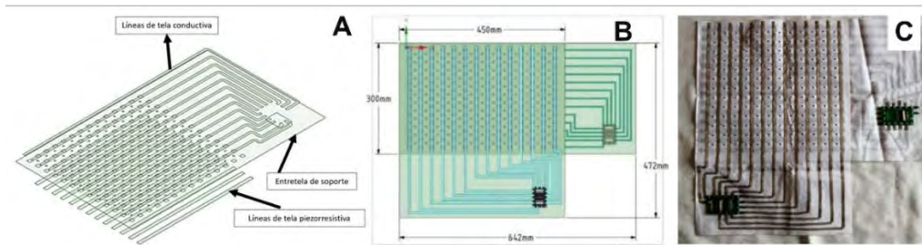
Figura 9. Diseño del sensor de distribución de presión (también llamado cojín): A) Componentes de la capa superior del sensor. B) Diseño en CAD de la distribución de filas y columnas del sensor. C) Sensor fabricado luego de corte láser y plastificado
