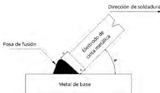
Figura 7. Dirección de la soldadura
