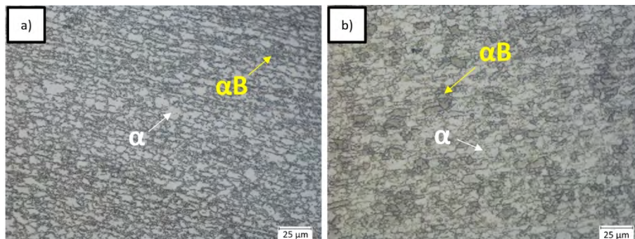
Figura 5. Metal base acero FB 700, a) 500X, Nital 2% - 9 s, b) 500X, Picral 2% - 7 s, Metabisulfito de sodio - 15 s con gotitas de HCl
