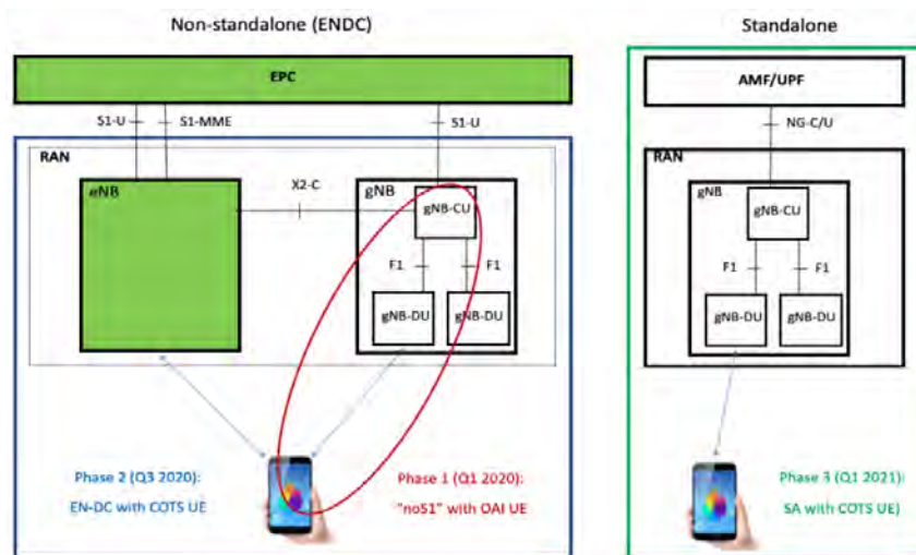
Figura 2. Esquema 5G NSA y 5G SA [19]
