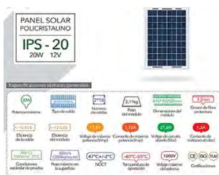
Figura 10. Panel Fotovoltaico Policristalino de 20W-12V [10]
