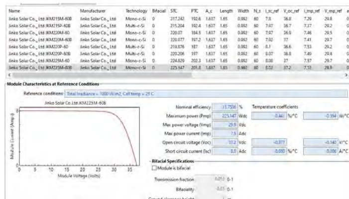
Figura 8. Características SAM [8]
