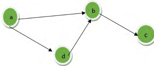
Figura 3. Grafo dirigido
