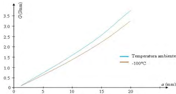
Figura 10. Comportamiento de los valores de G a temperatura ambiente y a -100\text{ }^{\circ}\text{C} . Esfuerzo plano
