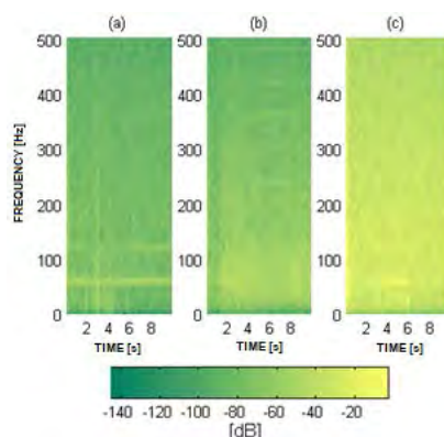
Figura 9. Espectrogramas comparativos, sujeto 3, señal diferencial 35, (a) inicial, (b) filtro RRLS, y (c) filtro ACC
