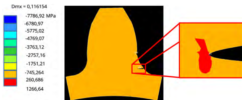
Figura 20. Grieta extendida a 10 mm de manera perpendicular a la línea de máximo esfuerzo principal
