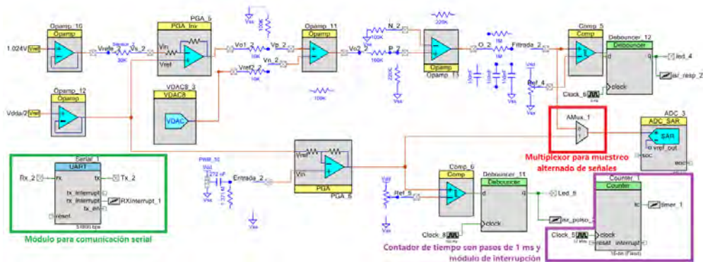
Figura 7. Integración de la etapa de acondicionamiento de los dos sensores usados. Se usaron cuatro amplificadores operacionales, dos PGA, dos comparadores con histéresis, un DAC, dos circuitos antirrebote, un mux analógico, un ADC-SAR de 12 bits, un contador y un módulo UART
