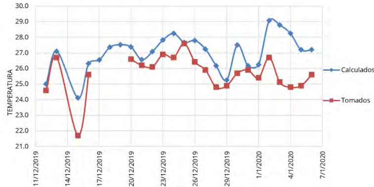
Figura 11. Comparación de temperatura superior del Tablero puente Tizón al amanecer
