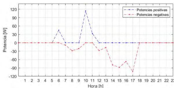
Figura 21. Perfil de potencia sistema de almacenamiento en un día
