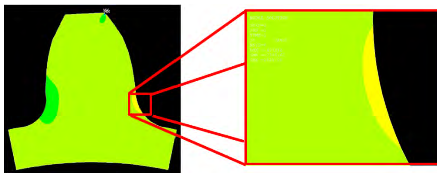
Figura 5. Campo de isopáquicas obtenido debido a la carga sobre el círculo exterior del diente del engrane
