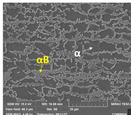
Figura 6. Micrografía obtenida por MEB a 4kX del metal base, se observan granos de bainita y una matriz ferrítica
