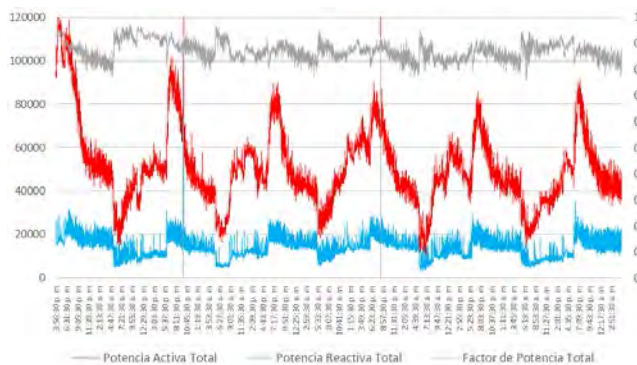
Figura 7. Potencia Activa, Reactiva y FP Subestación 4
