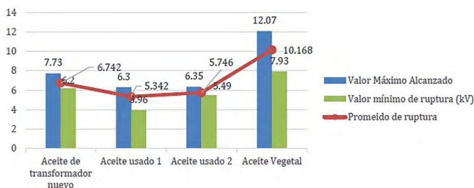
Figura 11. Gráfica de valores promedio vs valores máximos y mínimos basados en el estándar ASTM D1816
