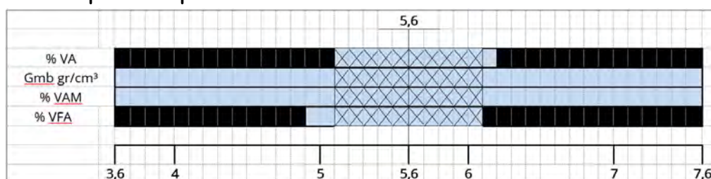
Figura 10. Determinación gráfica del rango óptimo de bitumen para el diseño Marshall
