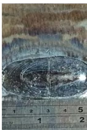
Figura 15. Aspecto exterior del cordón de soldadura - Prueba 2
